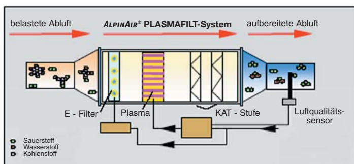
Abb.: ALPINAIR® PLASMAFILT System - Abluftreinigung
