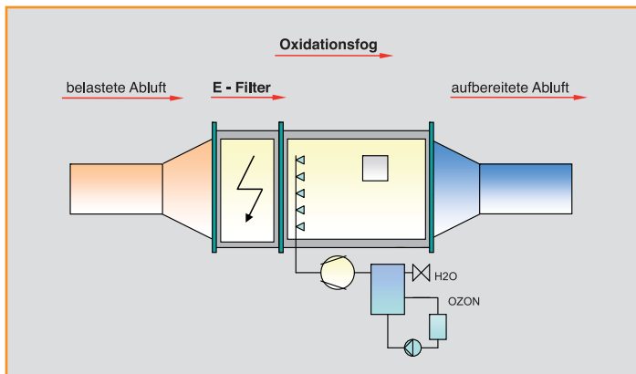
Abb.: Oxidationsfog - Geruchslösung
