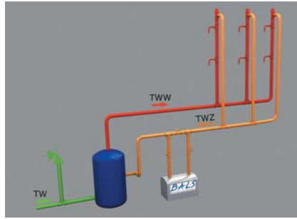
Abb.: Einbauschema BALS Liquid
