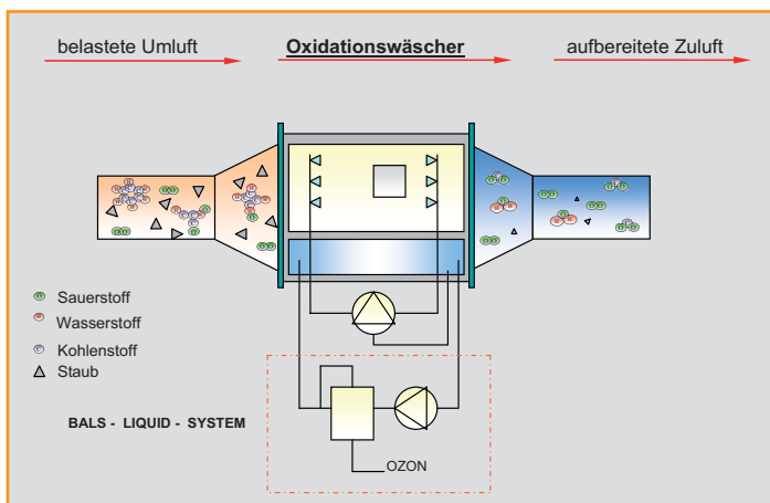
Abb.: Oxidationswäscher - Geruchslösung
