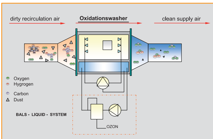
Fig.: Oxidationswasher - odor solution
