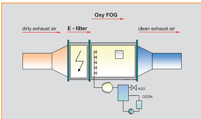
Fig.: Oxy Fog - odor solution
